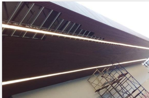
TRABAJOS DE MODERNIZACIÓN DEL TECHO E ILUMINACIÓN LED EN EL EXTERIOR DEL ÁREA DE ARRIBOS DEL AEROPUERTO INTERNACIONAL LA AURORA.
